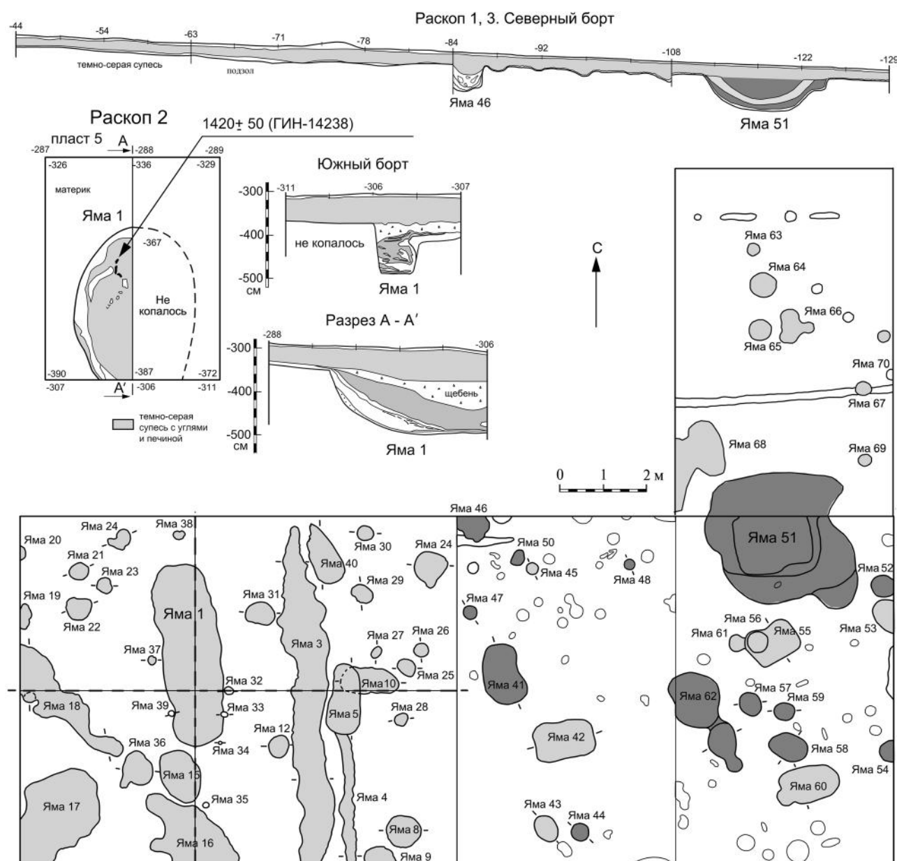
Рис. 4. Планы раскопов на селище Хотяжи 1. Темно-серым цветом показаны ямы с лепной керамикой; светло-серым — с круговой керамикой.
