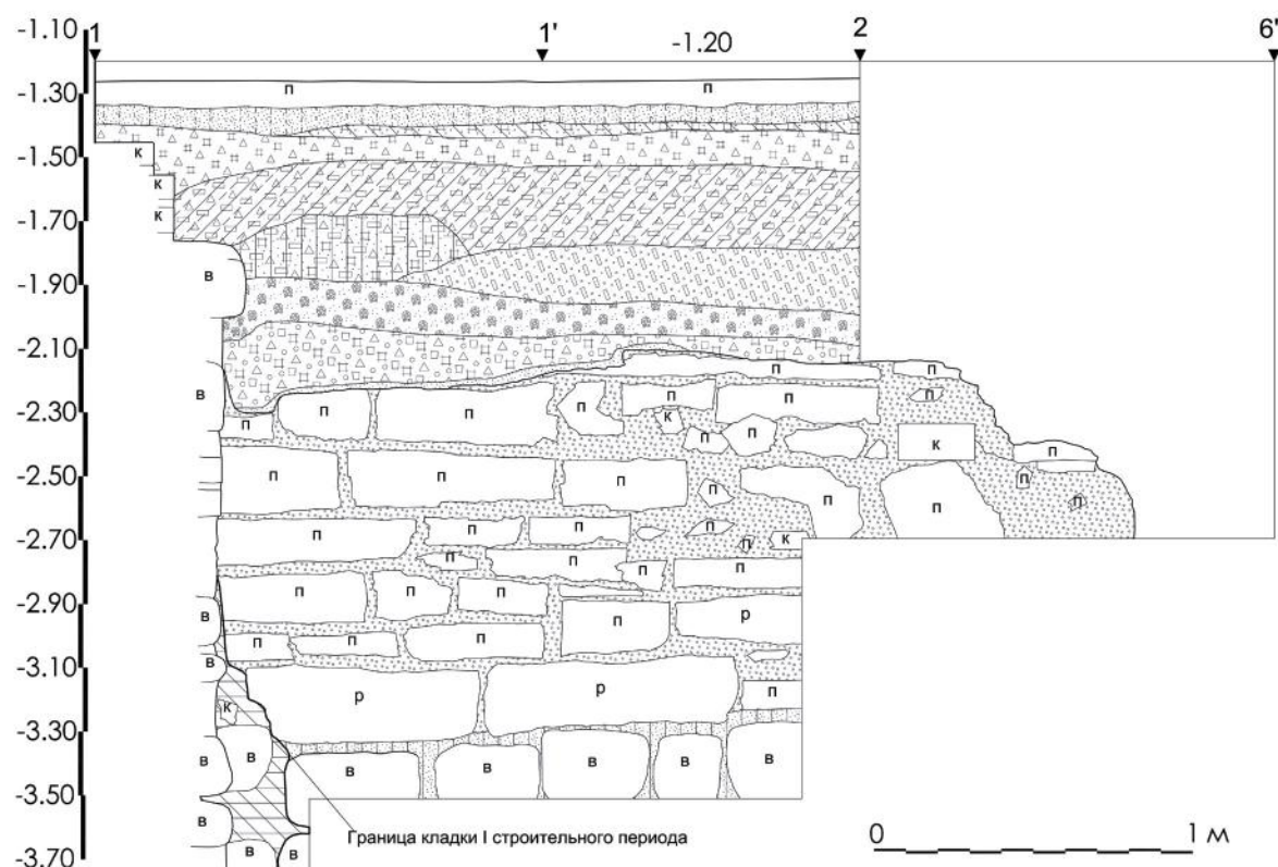
Рис. 5. Воскресенская церковь Деревяницкого монастыря, 1335 г. Южная плоскость южной стены западного притвора. Чертеж Т.В. Силаевой, И.В. Антипова, Д.Д. Ёлшина.
